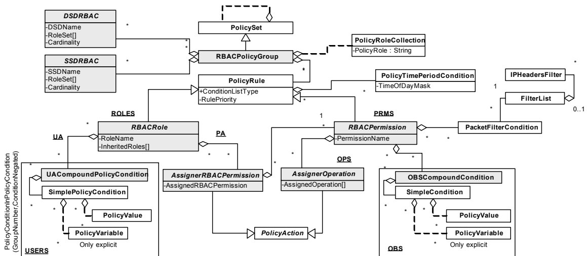
Figura 4.1 – Visão Geral do Modelo de Informação – RBPIM (revisado)
