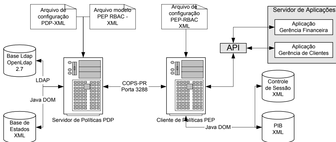
Figura 6.6 – Arquitetura de Implementação do Protótipo
