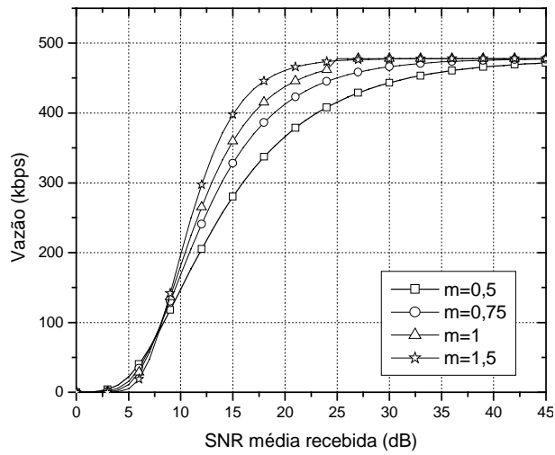
Figura 3.3: Desempenho do pacote DM5
