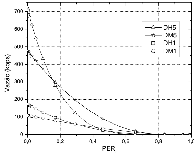
Figura 3.12: Vazão \times PER_r para m = 1,5
