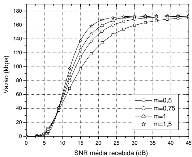
Figura 3.4: Desempenho do pacote DH1
