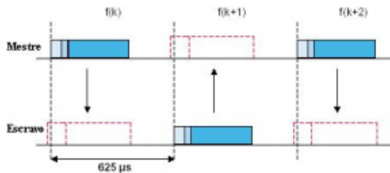
Figura 2.5: TDD (adaptado de [BLU01a] )
