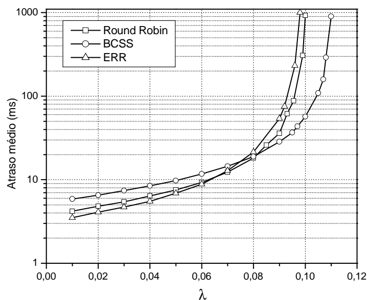
Figura 5.5: Atraso médio para d = 7m
