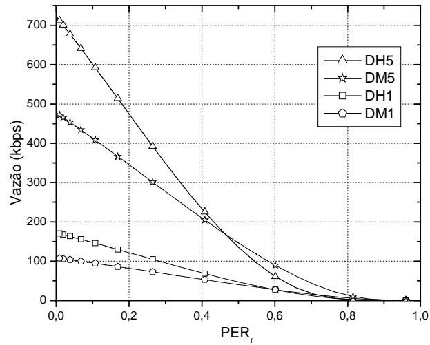
Figura 3.8: Vazão \times PER_r para m = 0,5
