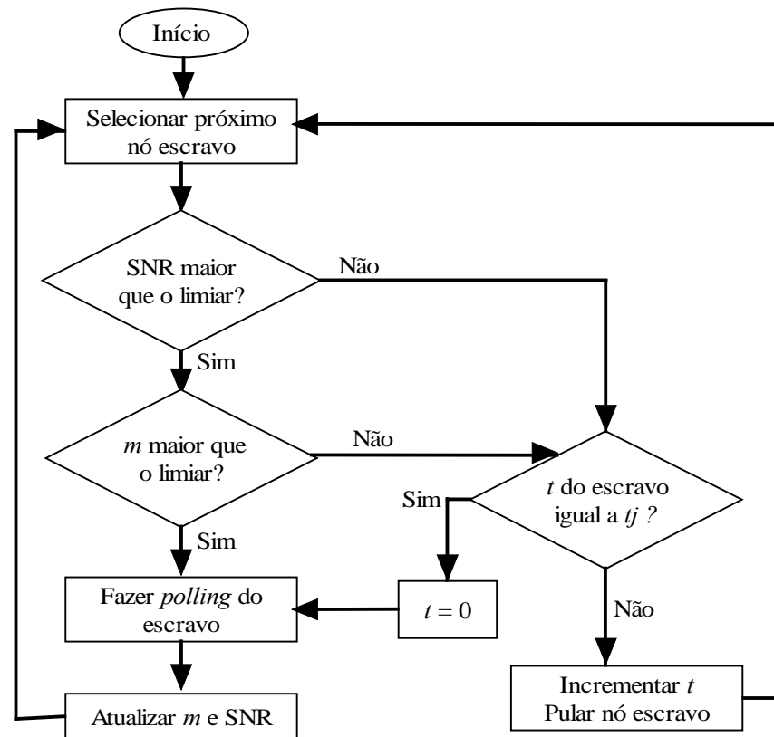
Figura 5.1: Algoritmo BCSS
