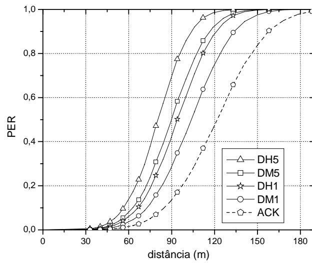
Figura 3.17: PER \times distância, m = 1,5 , \eta = 4
