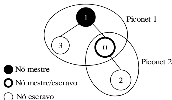
Figura 4.3: Topologia da scatternet para o primeiro exemplo
