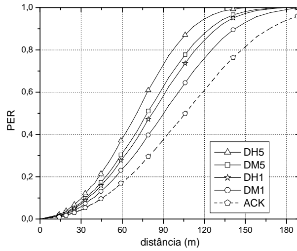
Figura 3.15: PER \times distância, m = 0,5 , \eta = 4
