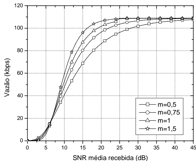
Figura 3.1: Desempenho do pacote DM1
