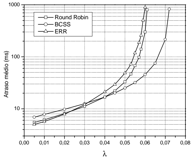
Figura 5.6: Atraso médio para d = 10m
