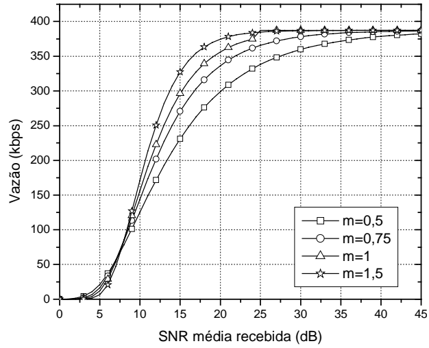
Figura 3.2: Desempenho do pacote DM3
