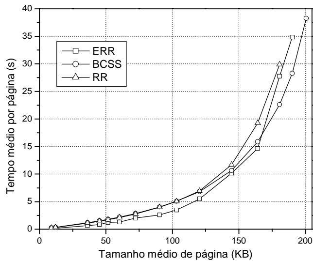
Figura 5.9: Tempo médio por página com 4 escravos
