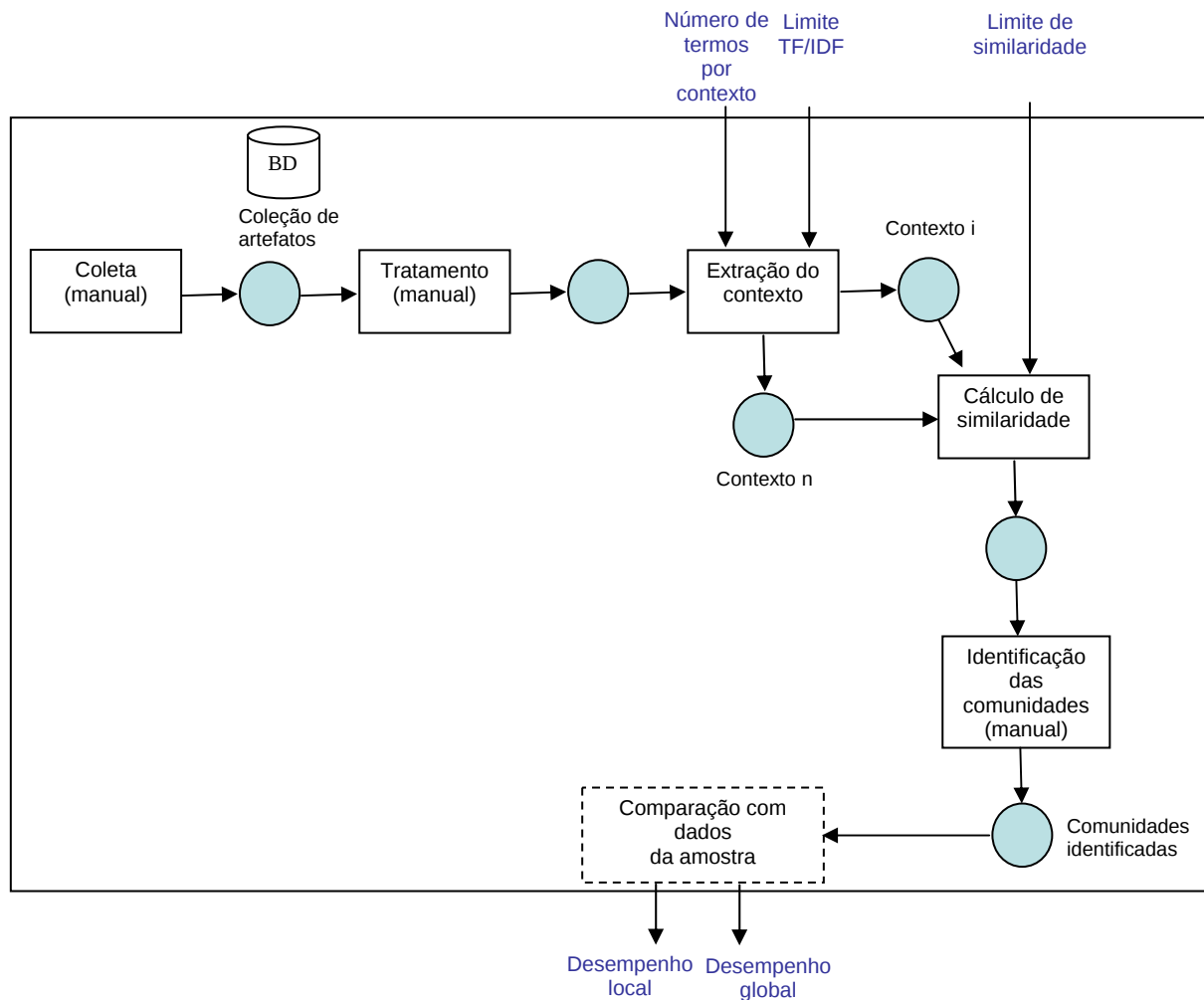
FIGURA 9 – Modelo experimental.
